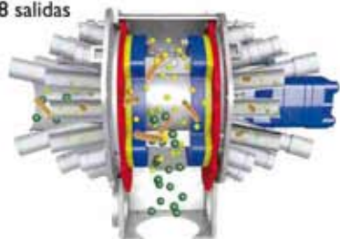
distribuidor 30/48 salidas
