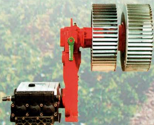
BOMBA DE PISTONES DE CERÁMICA
