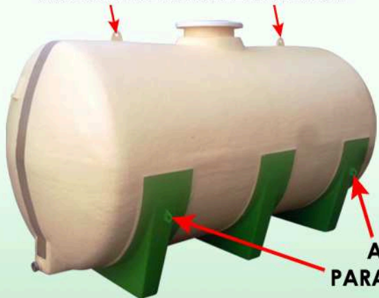
ARGOLLAS PARA ELEVACIÓN
