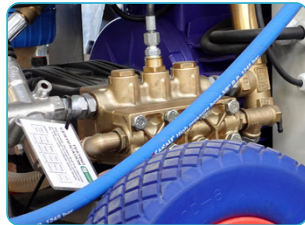
Cabezal de la bomba en latón.
