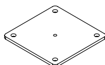
H020 - Chapa de anclaje espitar 200x200x8
