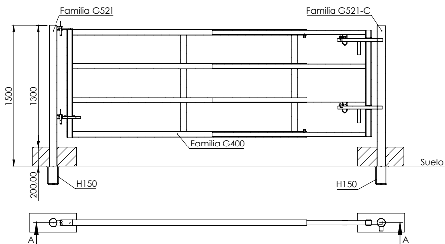
Tubo pilar G521
