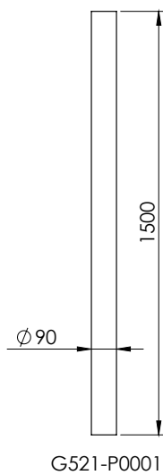
Tubo pilar G521
