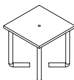
H200 - Chapa de anclaje encofrar 200x200x10
