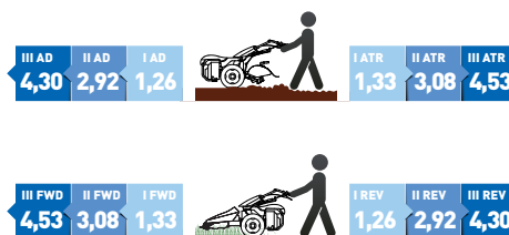
GRÁFICO VELOCIDAD EN KM/H CON RUEDAS 5.0-10
