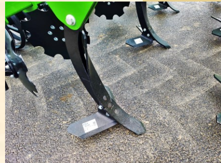
Reja, volteador y aletas
