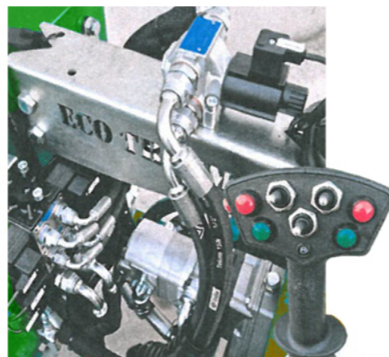
DISTRIBUIDOR ELECTROHIDRÁULICO CON JOYSTICK
